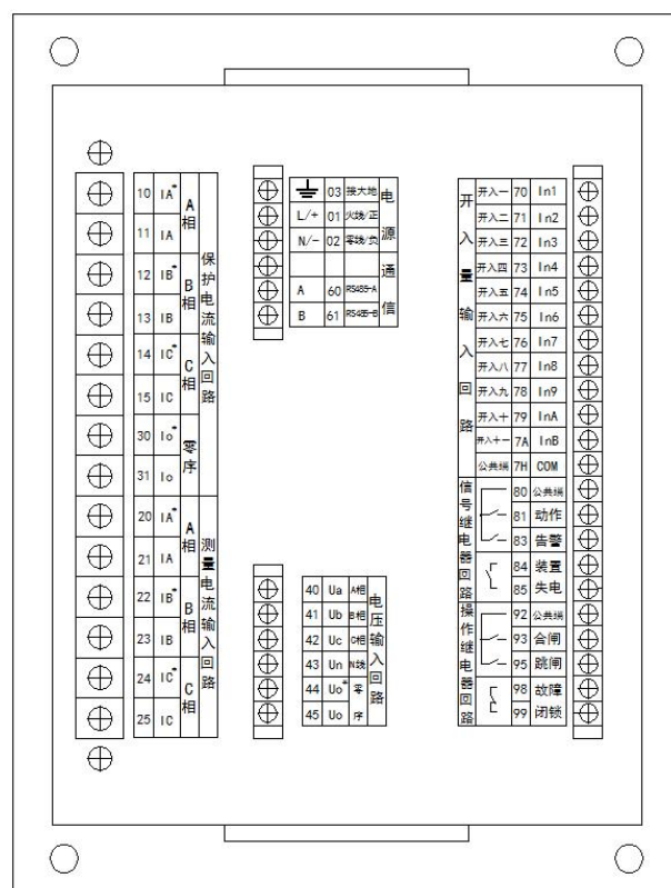
背视图
