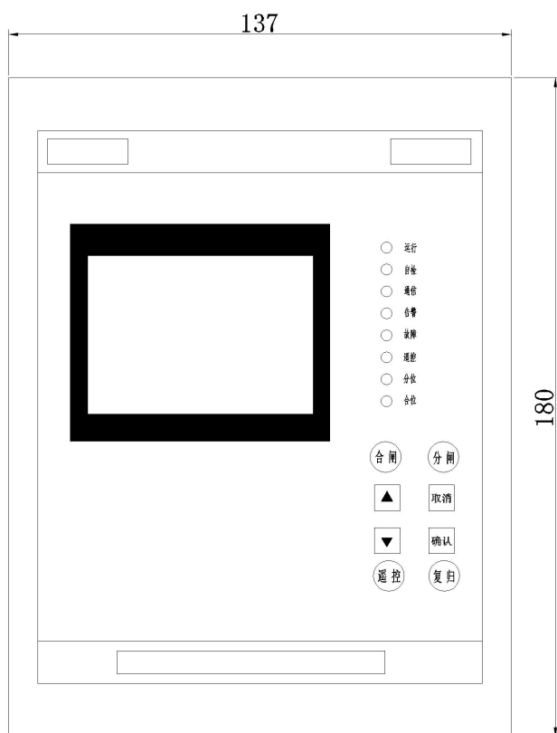
正视图
